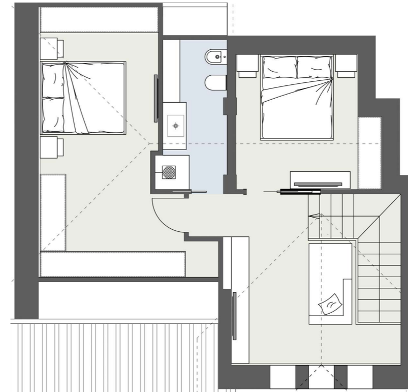
SOTTOTETTO MANSARDATO
